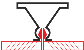
CLIP-IN SİSTEM TAŞIYICI
